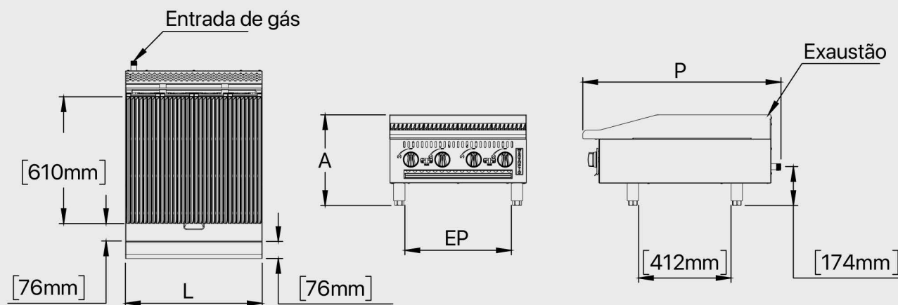
VISTA SUPERIOR
